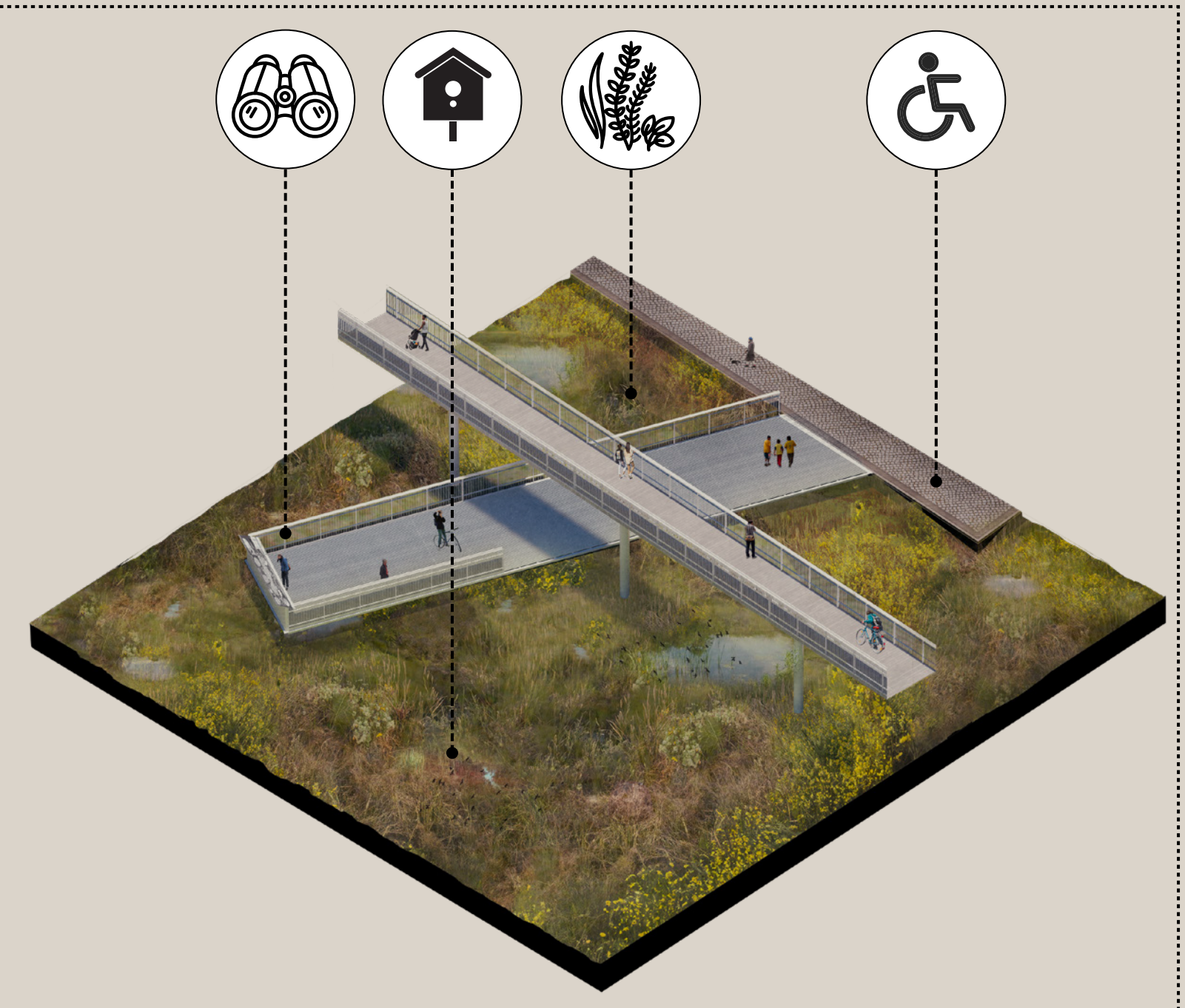
AXONOMETRICA / DETALLE PASARELA Y MUELLE SECTOR ESTANQUE CIRCULAR
